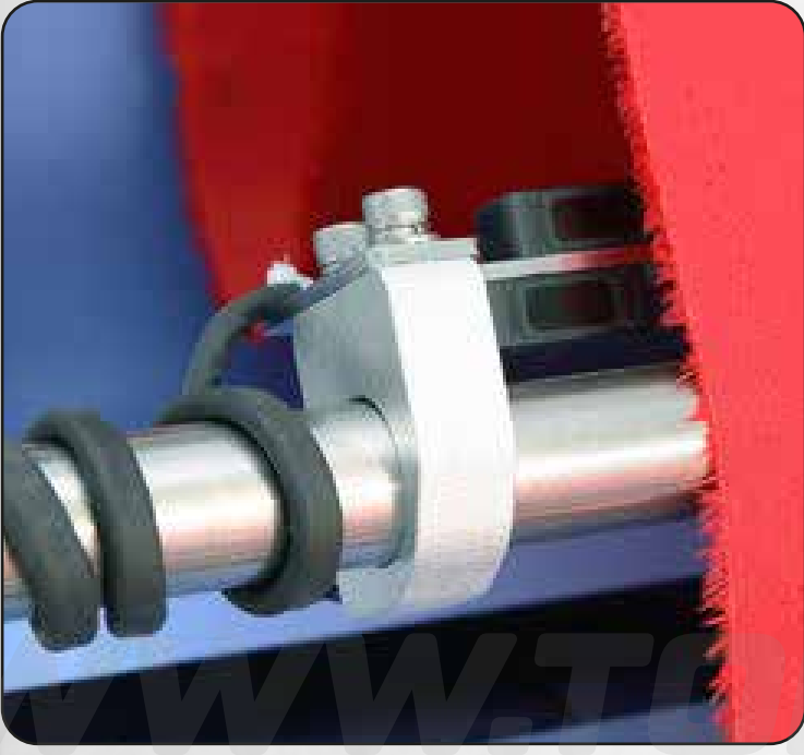
DISPOSITIVO DE BORDE AUTOMÁTICO DE OJO ELÉCTRICO
