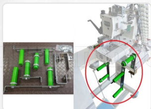
ROLLER PARA ELÁSTICO (PERMITE ENGOMAR LA CINTURA DE LA PRENDA SIN VARIACIONES)
