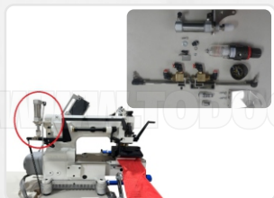
KIT LEVANTADOR DE PRENSATELA NEUMÁTICO (MEJORA LA PRODUCCIÓN EVITANDO LOS PROCESOS REPETITIVOS)
