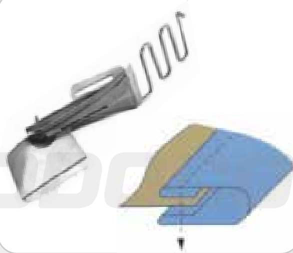
DOBLADILLADOR (MEDIDAS VARIAS)
